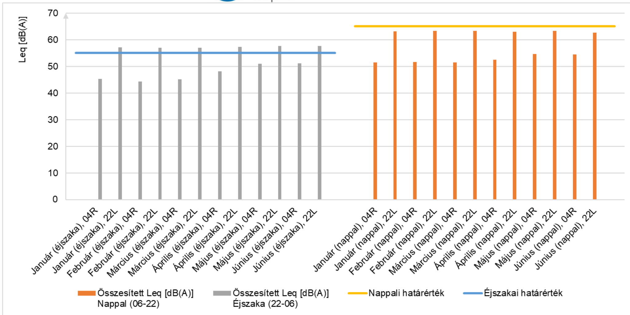
3. ábra: Egyenértékű A-hangnyomásszint ( L_{eq} [dB(A)]) változása havonta, zajmonitor pontonként összevetve az éjszakai és nappali zajszintre alkalmazott határértékekkel
